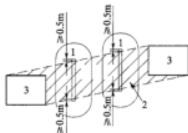
图 5.4.1-2 一字形防护土堤的平面防护范围
